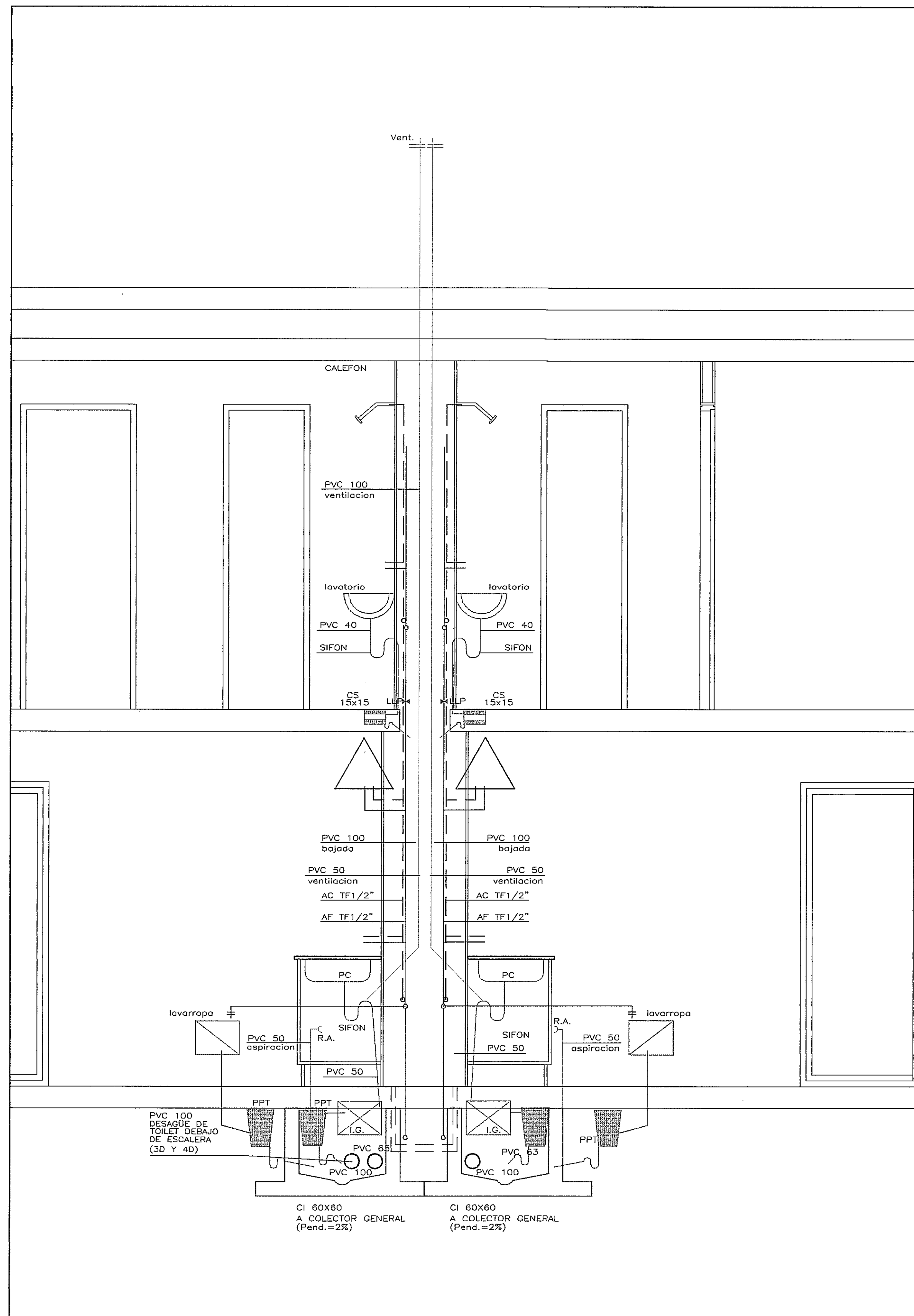
CORTE TRANSVERSAL DUCTO ESCALA 1:20
